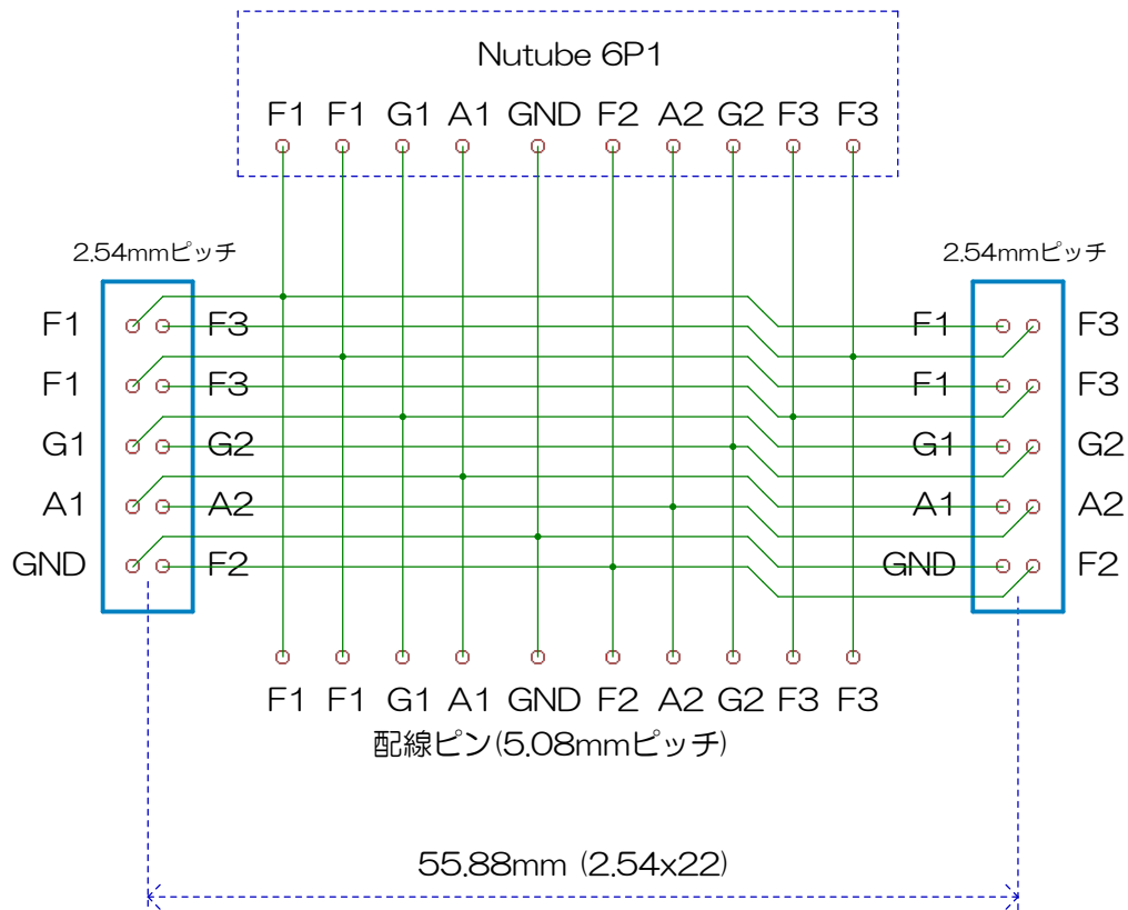
基板回路図
