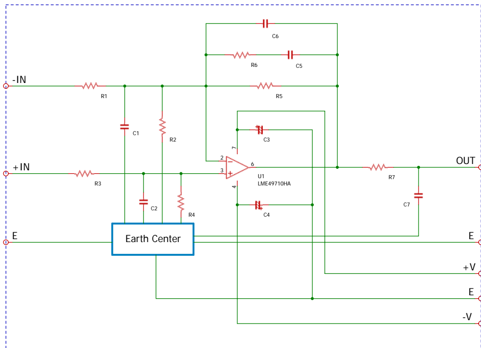
基板回路図
