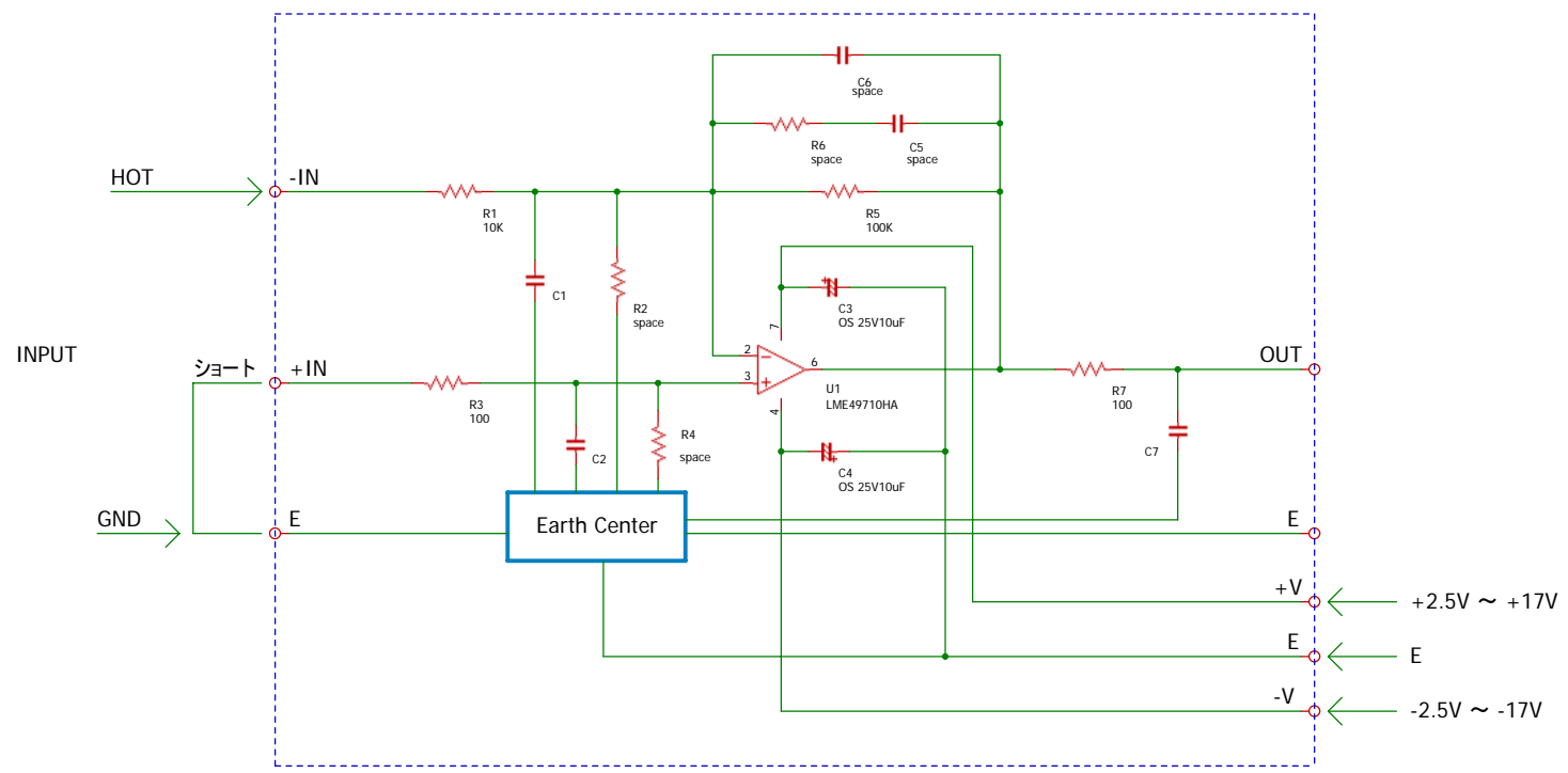
反転増幅回路図
