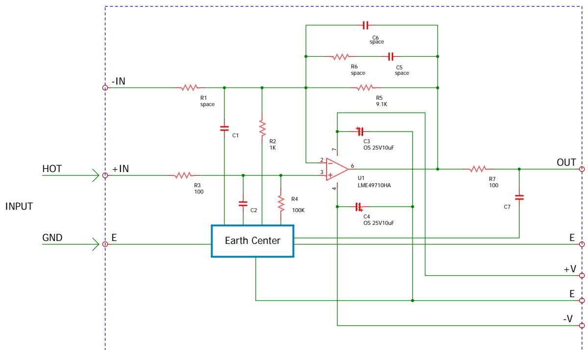
非反転増幅回路図
