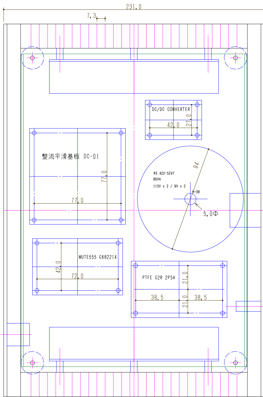
ヒートシンク (ケース内側より見た図)
