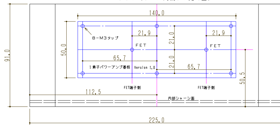
ヒートシンク (ケース内側より見た図)
